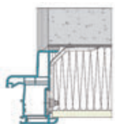
Doublage 100 mm
